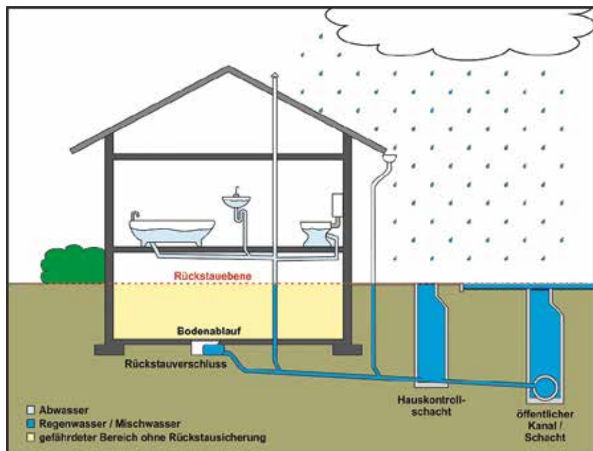
Schematische Darstellung der Rückstausicherung
