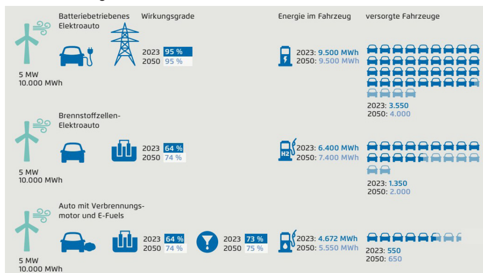
Abbildung 46: Effizienzvergleich verschiedener erneuerbarer Antriebsarten für einen Kompaktwagen mit einer Jahresfahrleistung 14.000 km/a (Agora Verkehrswende, 2023)
